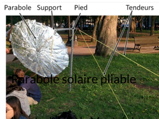
Parabole solaire pliable Low-tech Lab de Montréal, 2019. Voir fichier pdf ci-joint
