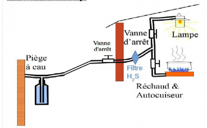
Annexe 6 : Schéma du réseau de biogaz
