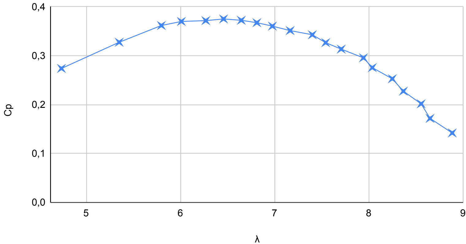
Cp en fonction de \lambda
