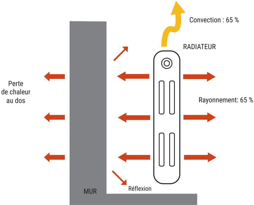
TRANSFERT DE LA CHALEUR DU RADIATEUR SANS RÉFLECTEUR
