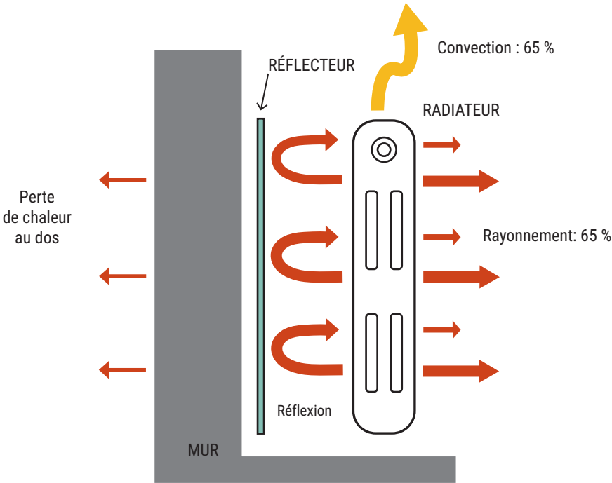
TRANSFERT DE LA CHALEUR DU RADIATEUR AVEC RÉFLECTEUR
