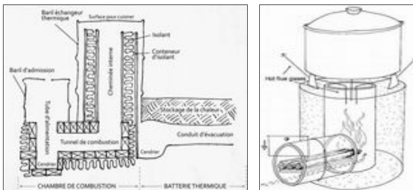
Rocket-Stove à gauche et cuisneur à bois à basse-consommation à droite.
