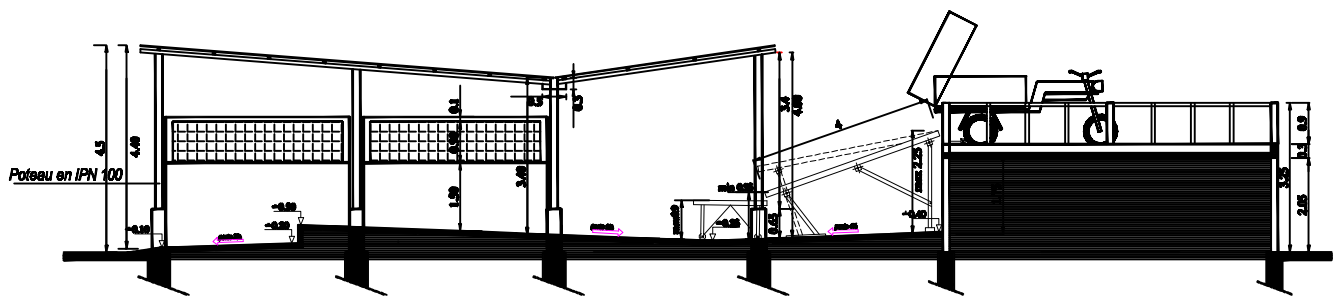
COUPE AA
