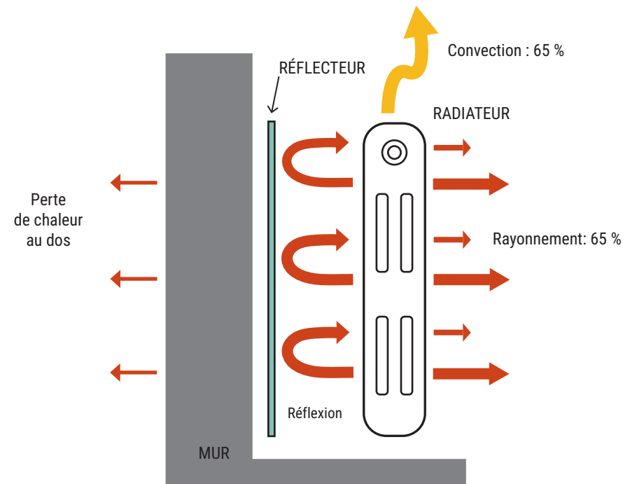
TRANSFERT DE LA CHALEUR DU RADIATEUR AVEC RÉFLECTEUR
